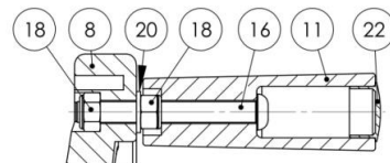
DOB RÖGZÍTÉS METSZETEM MŰKÖDTETŐ KERÉKKEL
