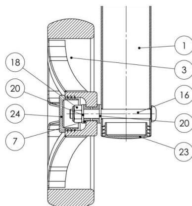
DOB RÖGZÍTÉS METSZETEM MŰKÖDTETŐ KERÉKKEL
