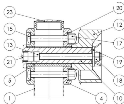
DOB RÖGZÍTÉS METSZETE
