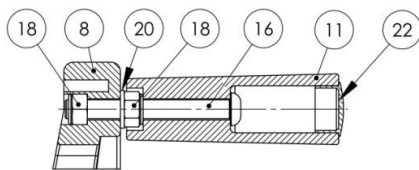
FOGANTYÚ RÖGZÍTÉS METSZETE
